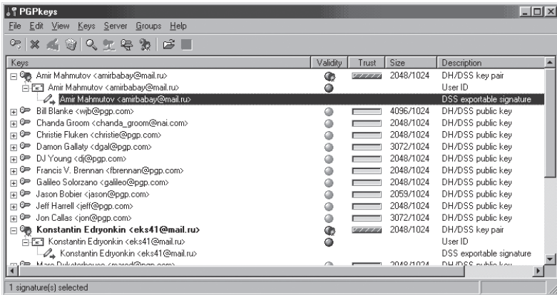
Рис. 2.7. Окно PGPkeys
